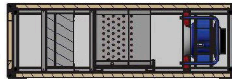
A-A ( 1 : 15 )
